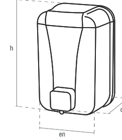
Kod :3424-S Standart Köpük Sabun Dispenserleri 500 cc. Siyah ABS + Siyah Görünüm Barkod : 8681451072642
